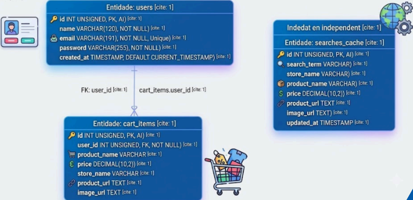
precio_db [cite: 1] – Diagrama Entidade-Relacionamento [cite: 1]
